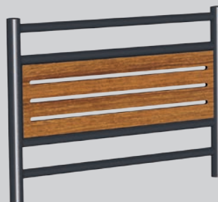
BR 21 - L 1 500 TÊTE BOMBÉE / PANNEAU COMPACT AJOURÉ (C21) LISSE SUPPLÉMENTAIRE BASSE (LI)
