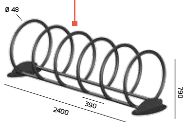
APPUI VÉLOS PV 200 / 6 Places A cheiller
