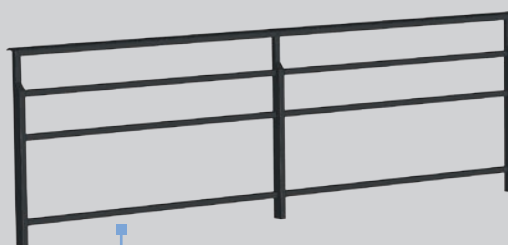
BR 42 C - L 3 000 2 LISSES PARTIE HAUTE SUPPLÉMENTAIRE (L41) **
